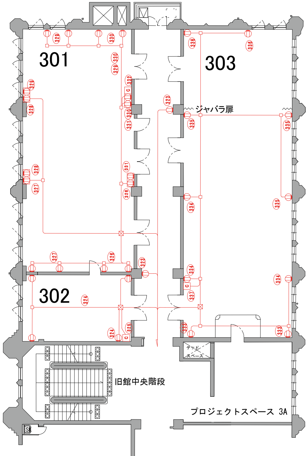
デザイン・クリエイティブセンター神戸 3階会議室 コンセント図
